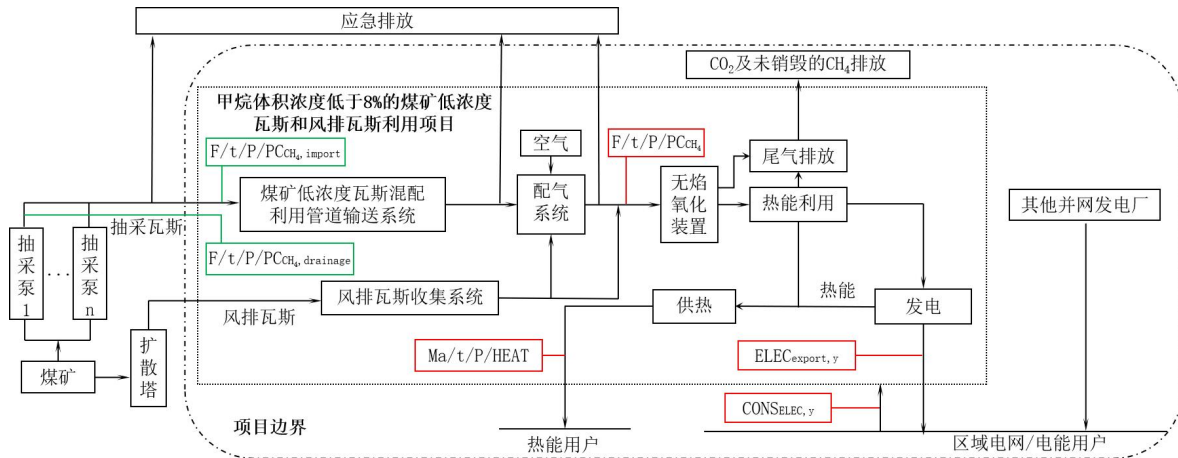
图 2 项目监测点布置示意图
