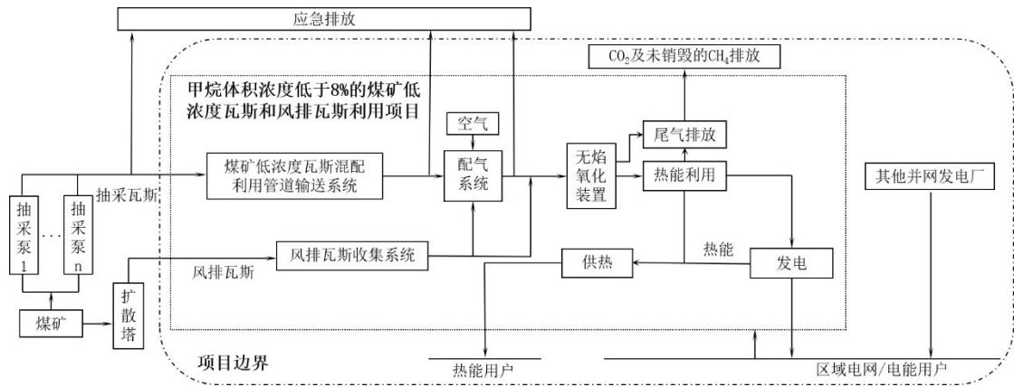
图 1 项目边界图
